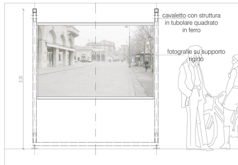
PARTICOLARE CAVALLETTO ESPOSITORE (ELEMENTO "A")
